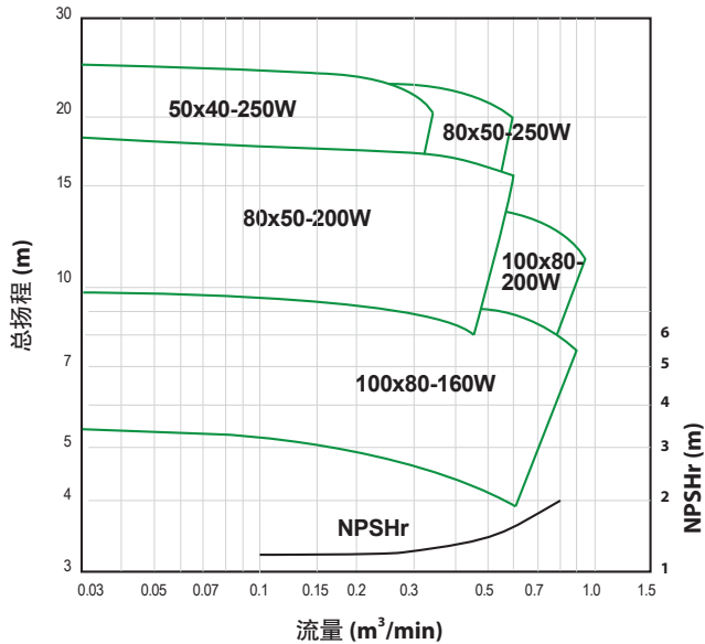
MTFO 2.2kW-5.5W 50 Hz, 4P- 1500RPM
