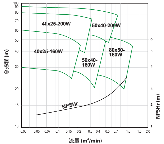
MTFO 2.2kW-5.5W 60 Hz, 4P- 1800RPM
