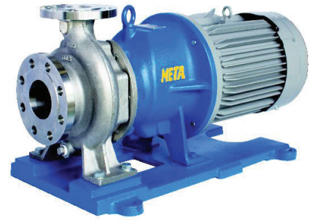
MTFO 3.7kW-22W 60 Hz, 2P- 3600RPM
